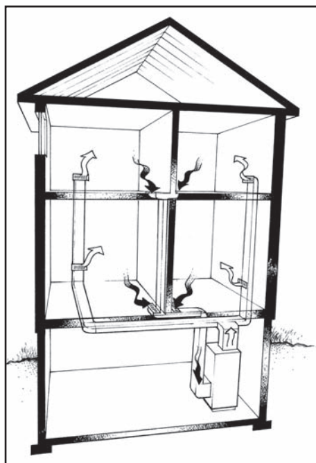
Figure 2 Distribution de l'air dans une maison
